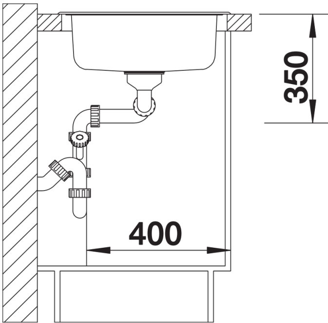
Oldalnézet
