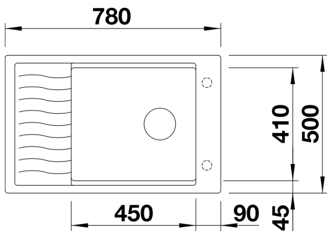
Felülnézet
